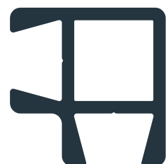
Pfostenmaße P60/E Ecke 60x60 mm
