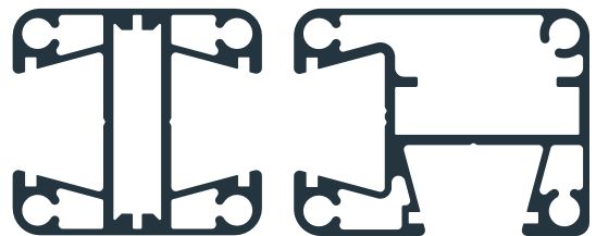
Pfostenmaße PV50 55x50mm
