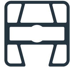
Pfostenmaße P60/1 Anfangs-/Endpfosten 60x60mm
